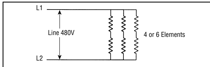
Figure 2 — 480 Volt Heaters
